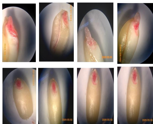
V1: Waha
