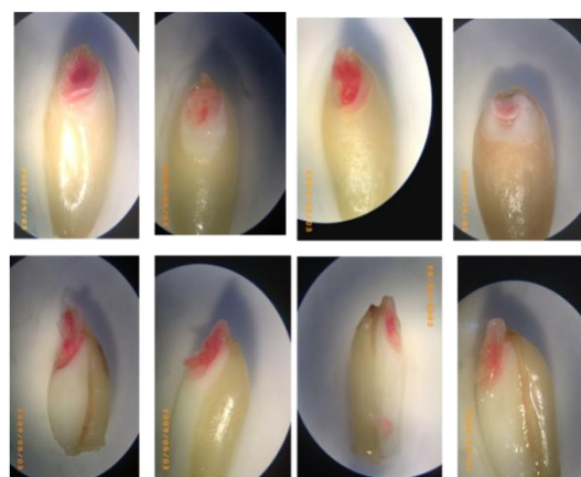
V3 : Stk/Hau/Heca-1
