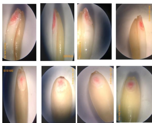
V2 : Gta/dur
