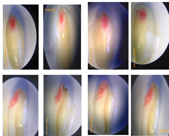
V4 : Ammar-8
