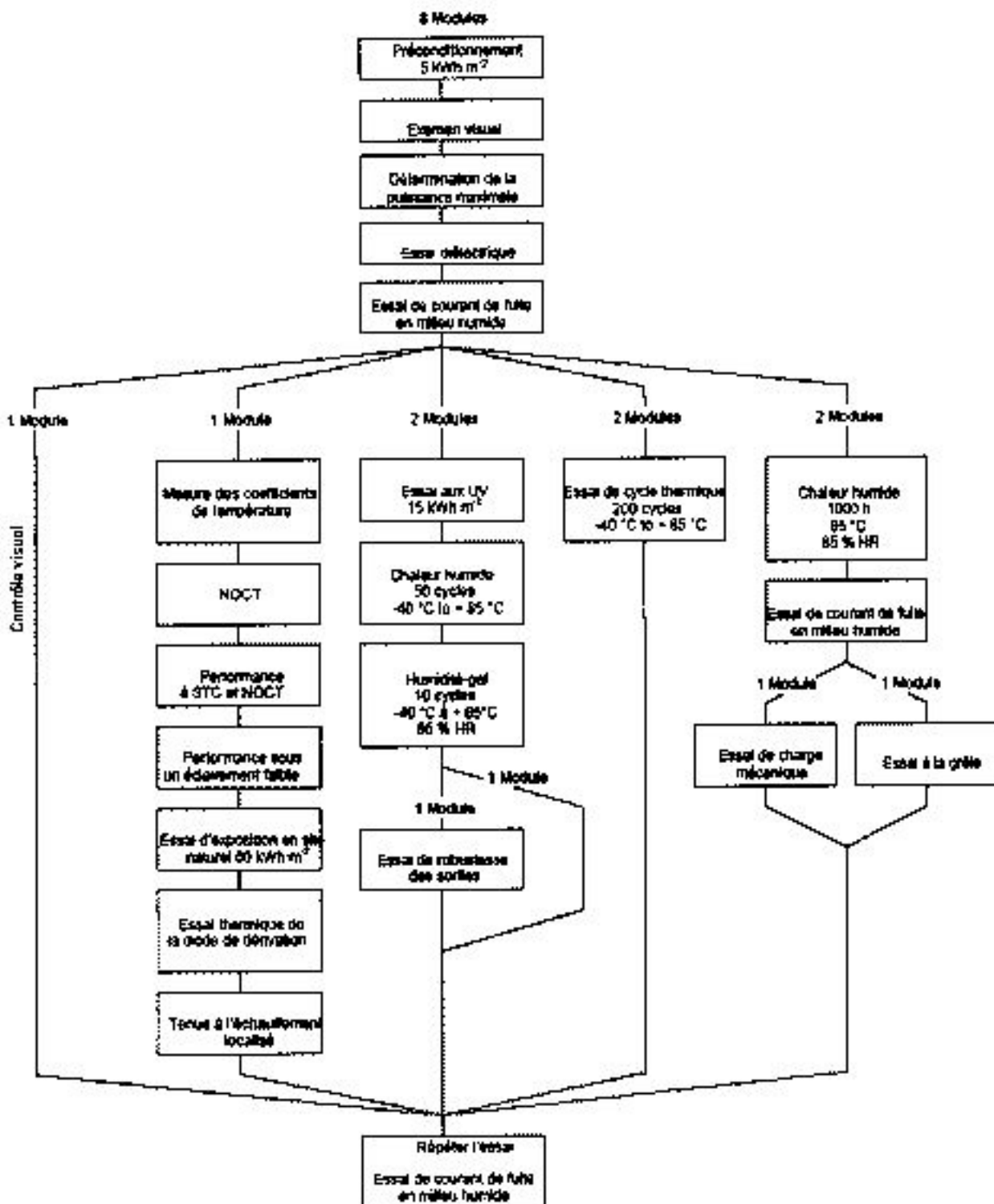
Déroulement des tests de qualification d'un module PV au silicium cristallin
